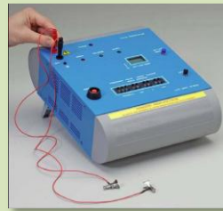
マウス用レスピレータ
